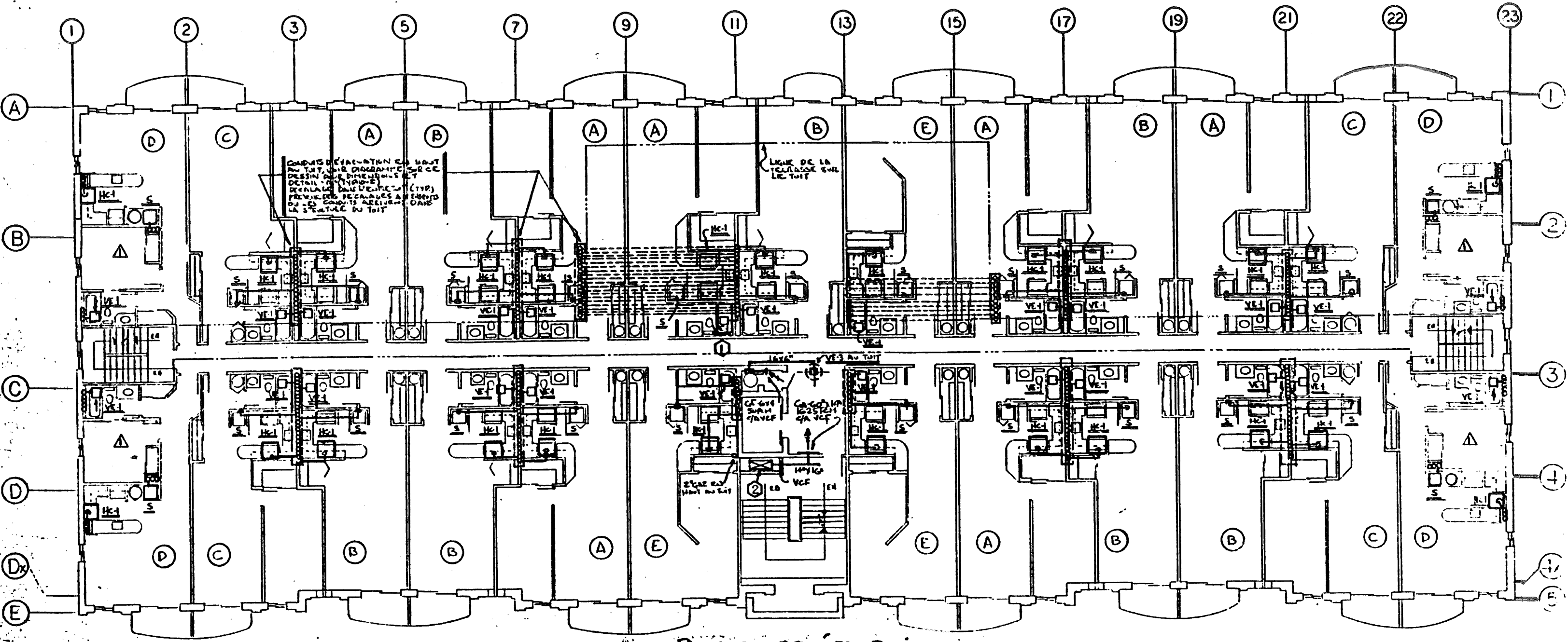
PLAN DU 3° ETAGE
